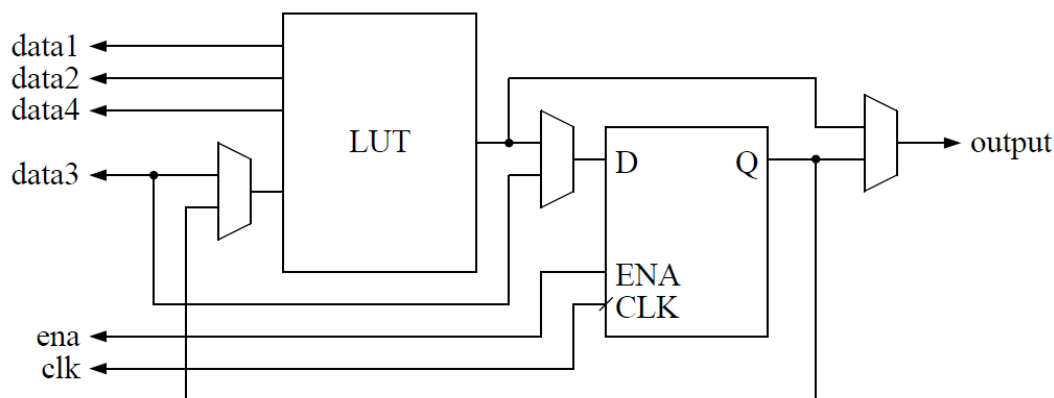
Рис. 6 – Структура LE – логического элемента FPGA Altera Cyclone II
