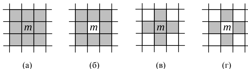
Рис. 3 – Некоторые типы окрестности радиуса r = 1 для ячейки m двумерного КлА: а) полная окрестность (окрестность Мура) б) квазиполная окрестность Мура в) окрестность фон Неймана г) неполная окрестность фон Неймана
